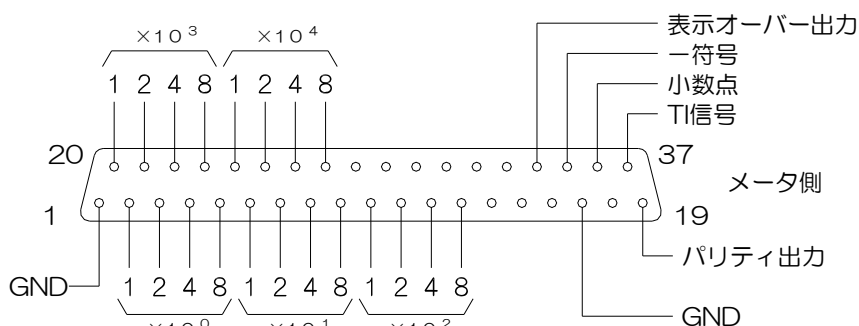
〔BCD出力ピン配置図（メータ側：D-Sub 37ピン メス）〕
