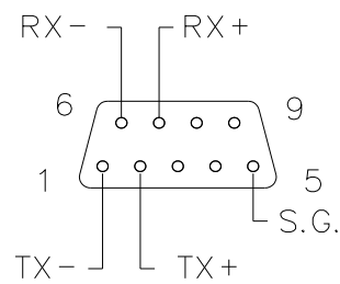
RS4W コネクタ
