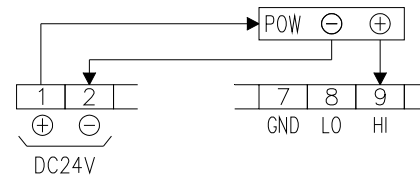
3線式センサ使用時 図5
