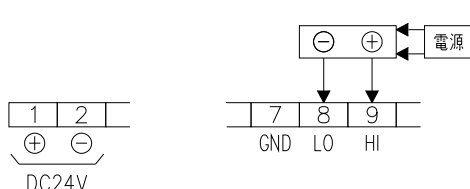
4線式センサ使用時 図6
