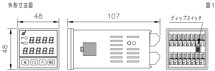
外形寸法図
