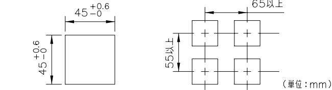
外形寸法図
