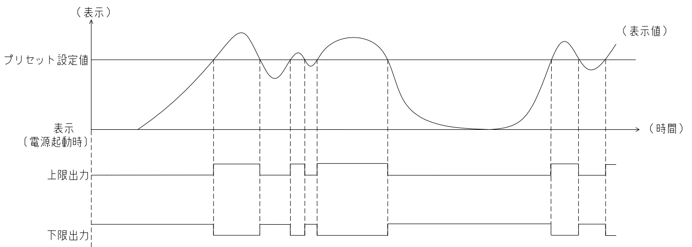
【警報出力タイミングチャート 参考図】
